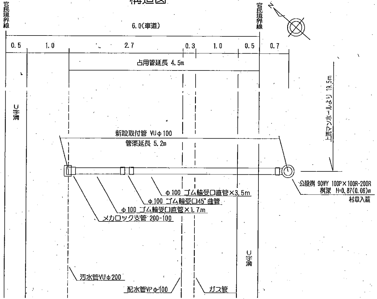
平面図 S=1:50
