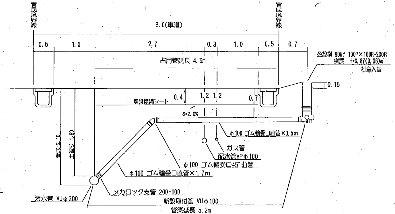
横断面図 S=1:50
