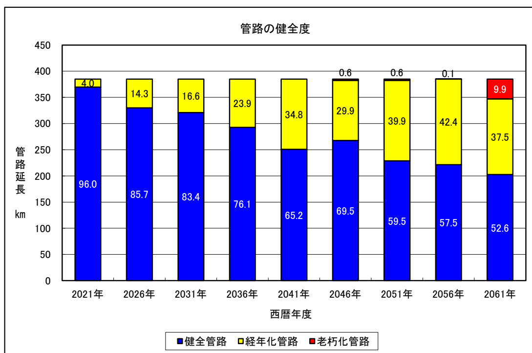
図 4-5 管路の健全度（更新基準で更新）
