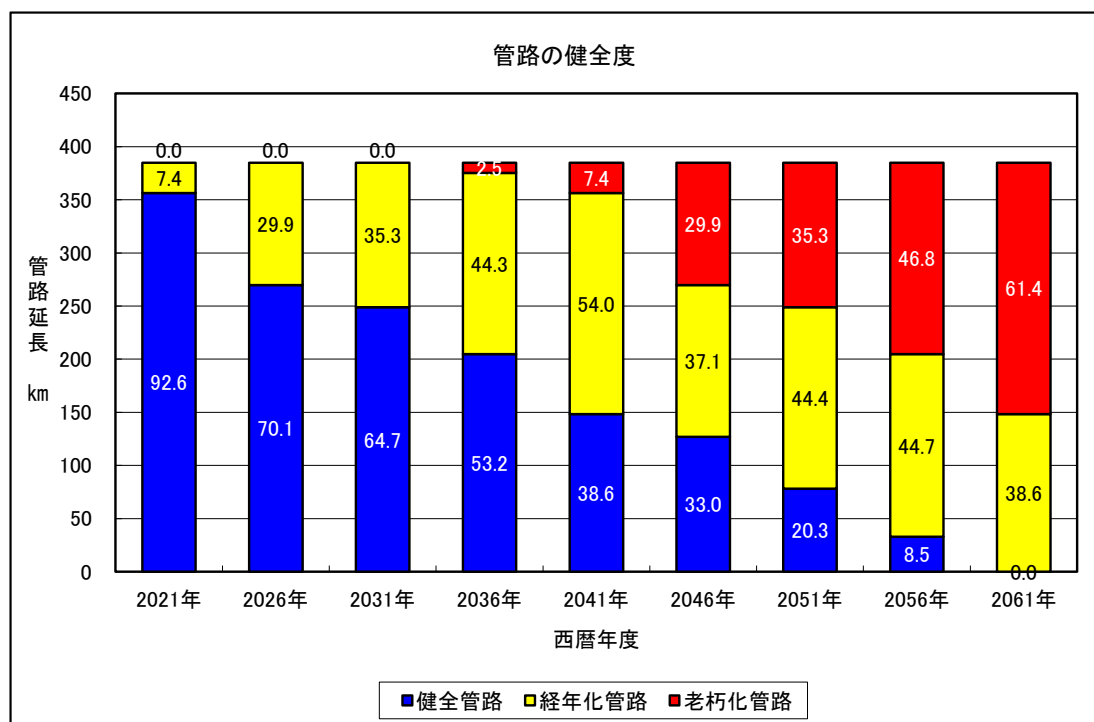
図 4-3 管路の健全度（更新なし）
