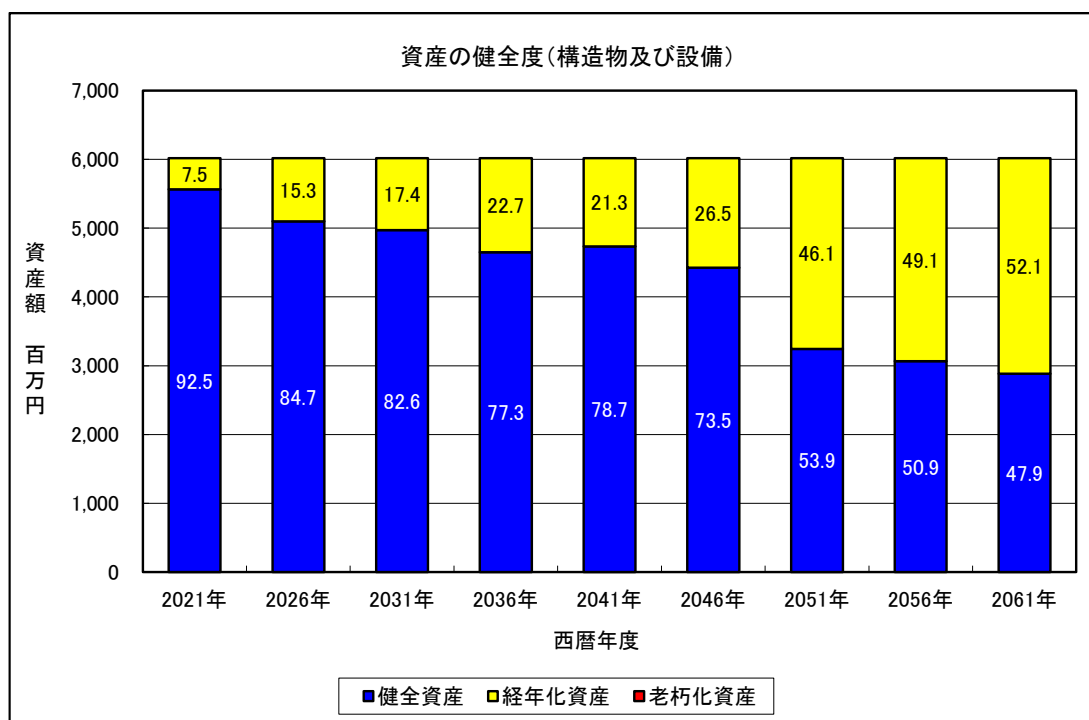
図 4-4 資産の健全度（更新基準で更新）
