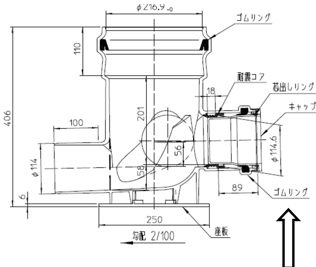
公共マス構造図
